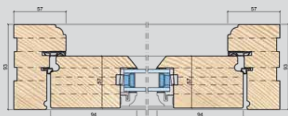
Jamb details
