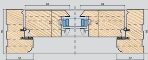
Jamb details
